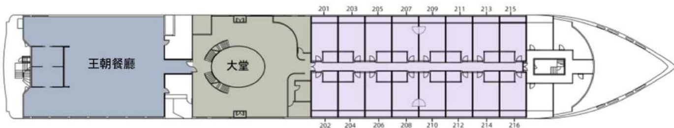
Deck 2 主甲板
