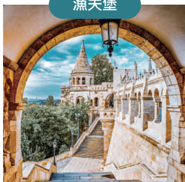
漁夫堡
